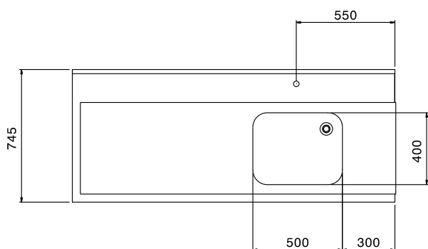
Boven aanzicht
